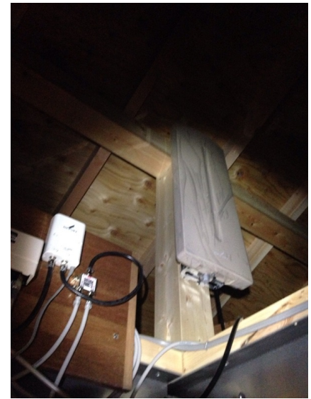
さいたま市岩槻区岩槻 松永住宅様物件 デザインアンテナ屋根裏工事
