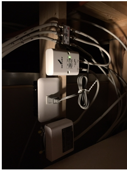
さいたま市岩槻区 コガネイハウジング様物件 5分配器 ブースター本体 ブースター電源部
